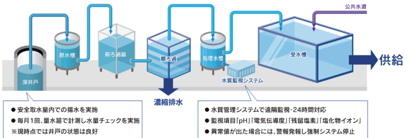
井戸水処理水槽 汲み上げた井戸水をB2Fプラント内の水槽に貯留。
