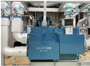
ターボ冷凍機 (冷熱)
